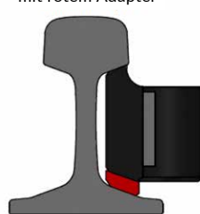
Vignol 54E2 mit rotem Adapter
